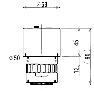
マイクログラフ 本体
